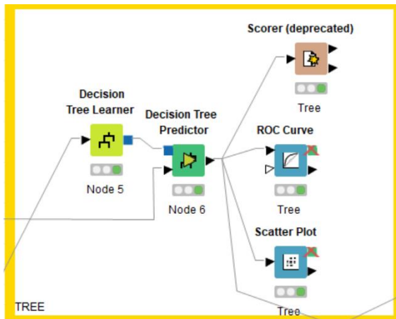
Figura 6. Diagrama de bloques del clasificador de árboles de decisión
