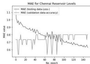
Fig. 5. Resultado del entrenamiento
