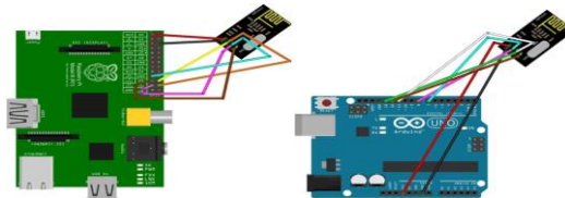
Figura 9. Conexión Raspberry Pi - Arduino
