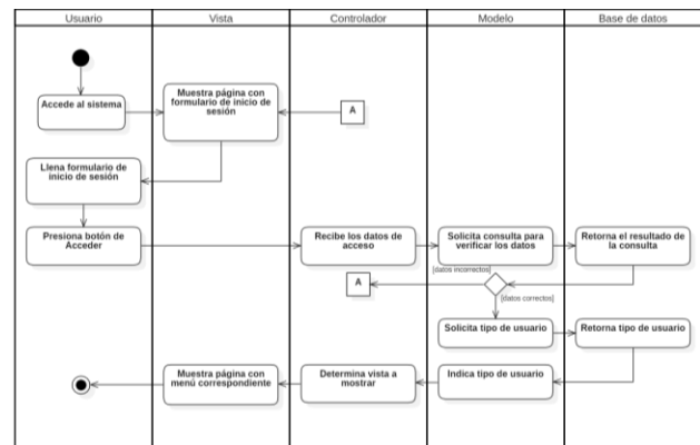
Figura 1. Diagrama de actividad del requisito F.N.1.
