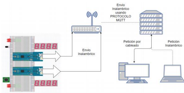
Figura 4. Estructura, protocolo y topología de comunicación del proyecto
