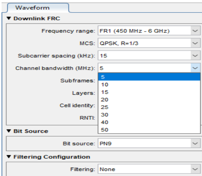
Figura No. 3: Anchos de banda del canal FR1 en Downlink
