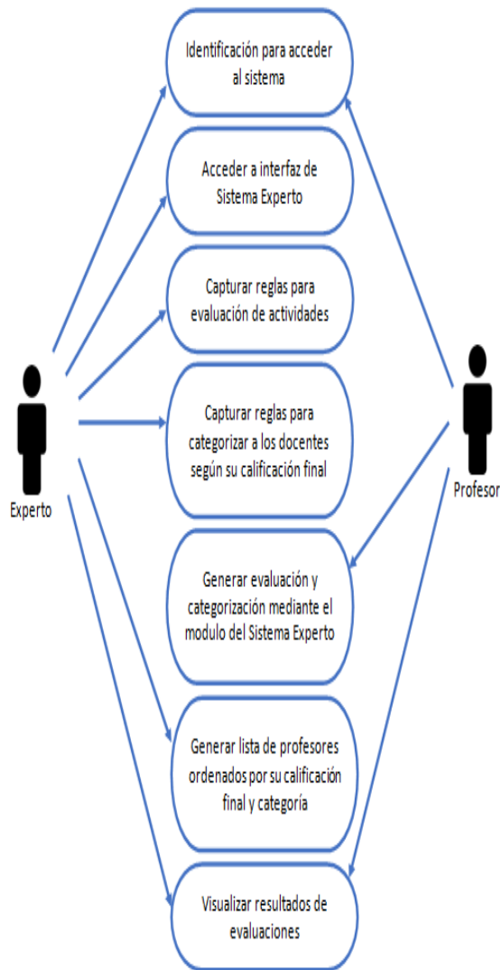
Figura 3. Diagrama de Caso de Uso de Sistema Experto
