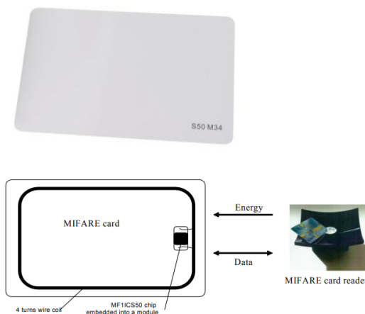
Figura 8. Tarjeta MIFARE S50
