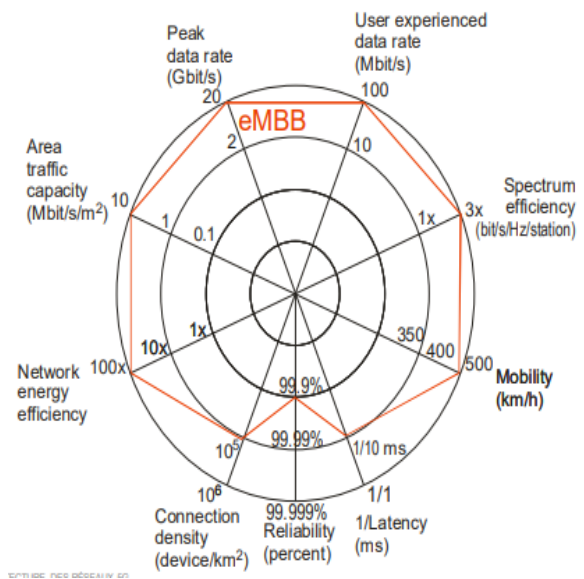
Figura No. 6. Ancho de banda mejorado eMBB de la 5G
