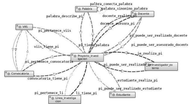
Figura 3. Diagrama de relaciones binarias de la ontología.
