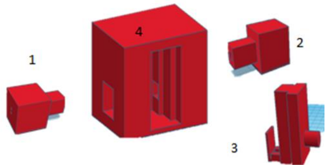
Figura 2. Diseño 3D de las partes del analizador del espectrofotómetro
