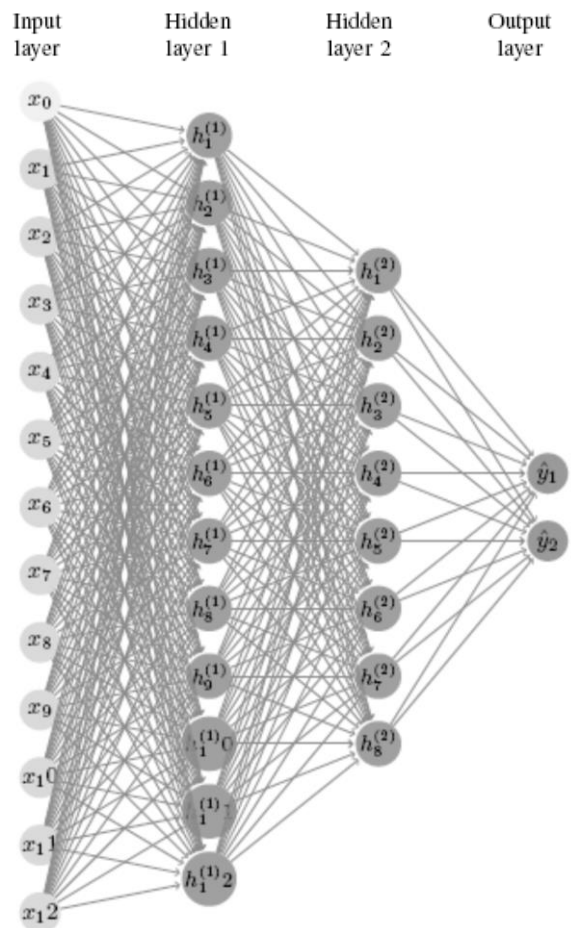
Figura 3. Modelo red neuronal.
