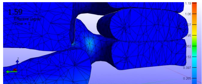
Figura 16. Vista del cruce de las mallas entre las vértebras y el disco, bajo la carga máxima soportada. Fuente: Elaboración propia.
