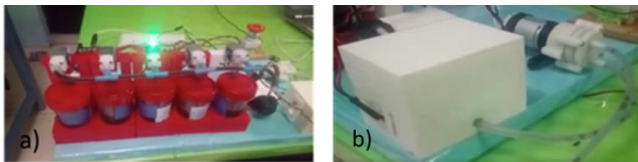
Figura 4. Imagen de las muestras analizadas, a) válvulas y la bomba de llenado, b) Analizador conectado con la bomba de desagüe y la bomba de llenado total mente sellado para disminuir interferencia del medio.
