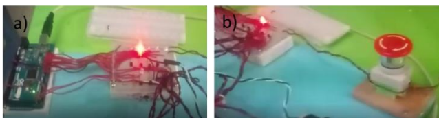
Figura 5. a) Placa con conexión a todos los instrumentos y con un bus de datos que conectan la placa Arduino (b) botón interruptor.
