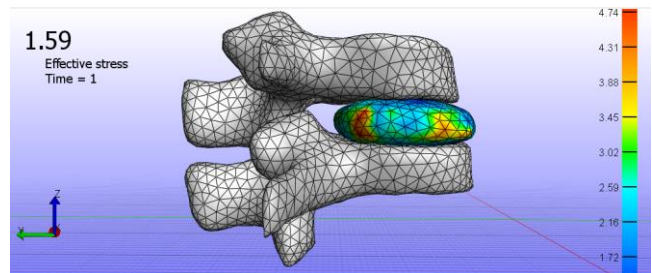
Figura 15. Vista lateral del cuerpo vertebral bajo la carga máxima soportada. Fuente: Elaboración propia
