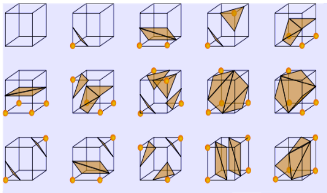
Figura 2. 15 combinaciones finales del algoritmo Marching Cubes [1]. Los puntos indican vértices que se han probado como "dentro" del objeto
