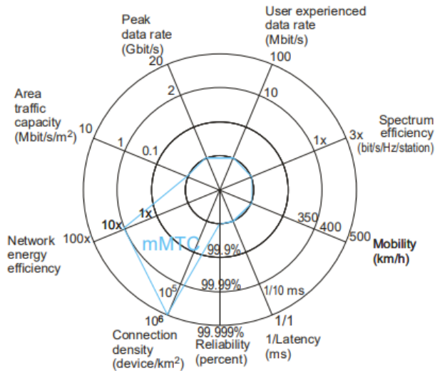
Figura No. 7. Aumento de la densidad con mMTC de la 5G
