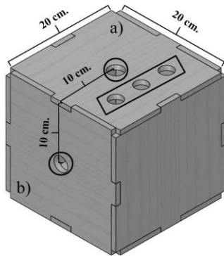
Figura 4. Diseño del box trainer. a) Cara superior, b) Cara lateral.
