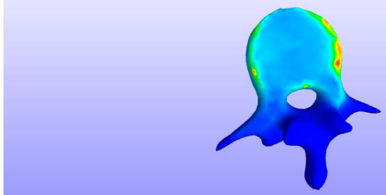
Figura 8. Vista inferior de la vértebra bajo una carga determinada. Fuente: Elaboración propia
