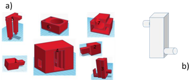
Figura 3. a) Diseño 3D del espectrofotómetro automático, b) Celda perforada y colocadas mangueras para el llenado y desagüe de la muestra.
