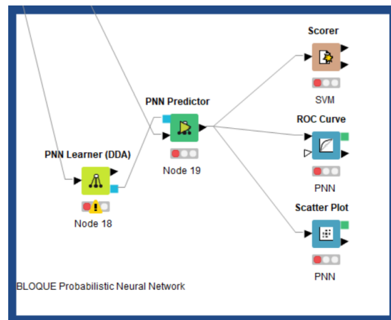
Figura 4. Diagrama de bloques del clasificador de red neuronal probabilística
