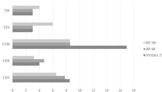
Figura 13. Grafica comparativa de plataformas embebidas. TIS: Tiempo inicialización de script, TES: Tiempo de inicio de ejecución de script, TAM: Tamaño, CER: Consumo energético en reposo, Consumo energético en ejecución.
