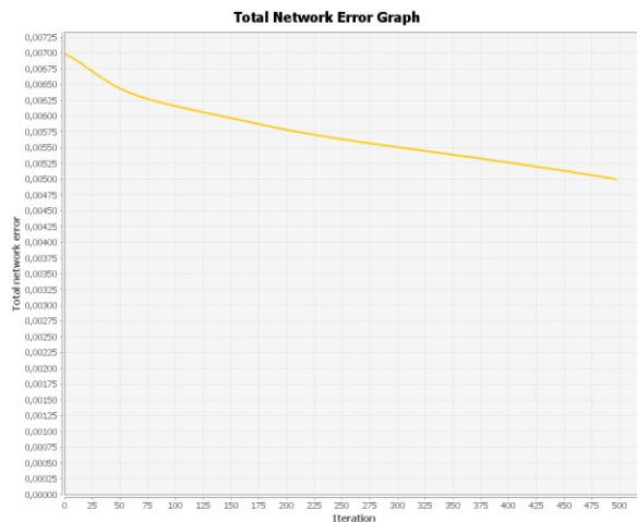
Figura 2. Comportamiento del error de entrenamiento en la tercera iteración de la RNA 7-14-10-8-1.
