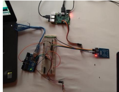
Figura 13. Comuniación netre Arduino y raspberry Pi
