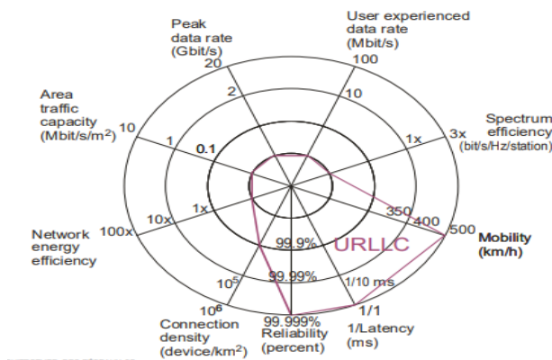
Figura No. 8. Reducción de latencia con URLLC de la 5G
