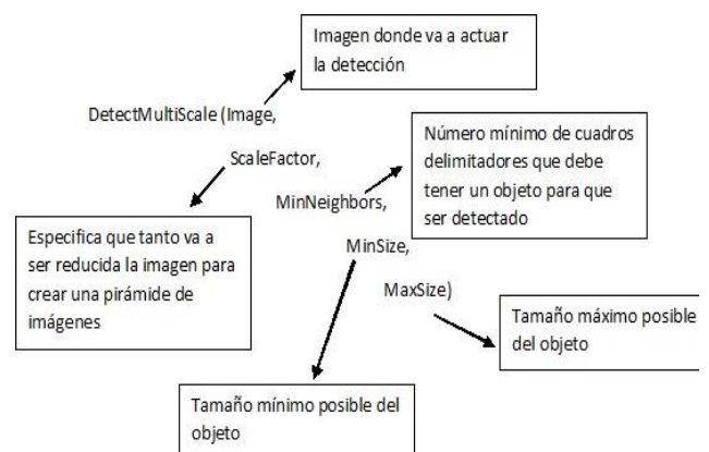
Figura 3. Estructura de DetectMultiScale. [7]
