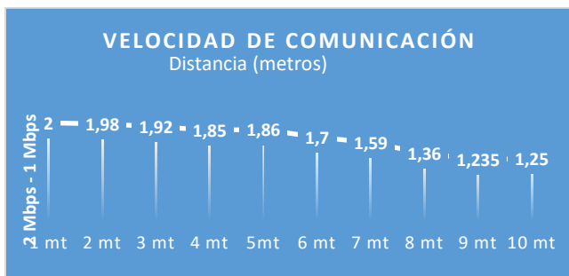
Figura 16. Velocidad de comunicación en línea de vista.
