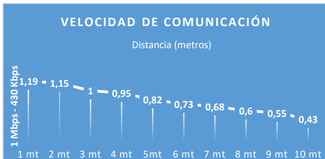
Figura 17. Velocidad de comunicación en línea de vista.
