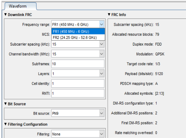
Figura No. 2: Canales FR1 Y FR2 5G del Downlink
