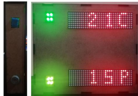
Figura 6. Prototipo electrónico con sensores de Monóxido de carbono y temperatura (PROMCAT)
