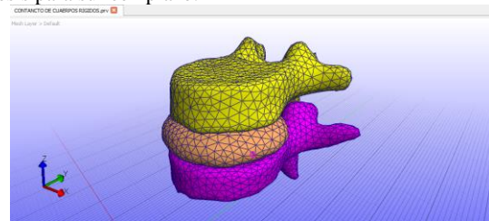
Figura 5. Estructura vertebral de L1 a L2. Fuente: elaboración propia.
